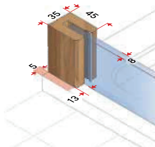
Průřez instalační situace na sprchovou vaničku
