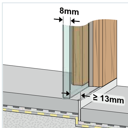
Průřez instalace na podlahu
