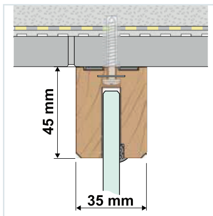
Průřez instalace profilu na obklad
