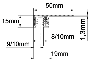
Podomítkový profil
