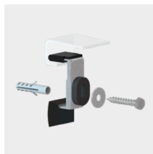
VANOVÉ KOTVY
