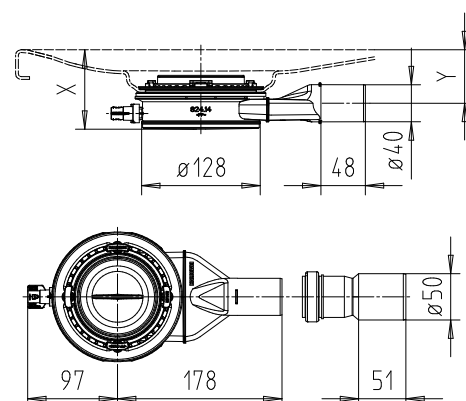
KA 120 PLOCHÁ
