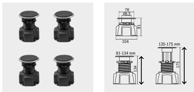
SADA MONTÁŽNÍCH NOHOU
