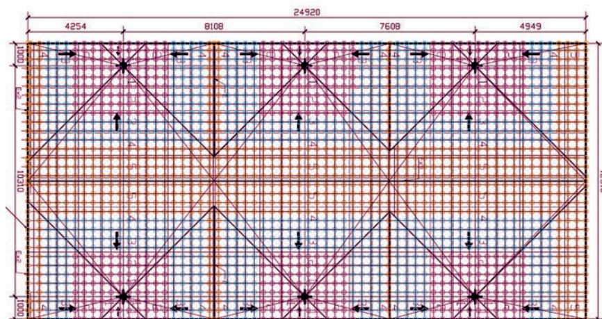
Příklad kladečského plánu a spotřeby terčů
