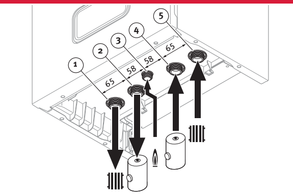
Připojení: systémový kotel, Zásobník TV
