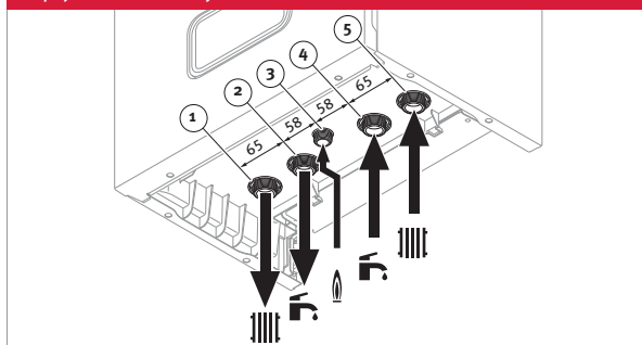
Připojení: kombinovaný kotel
