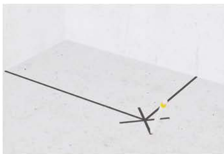
2. Přenést střed otvoru sprchové mísy na nosnou konstrukci
