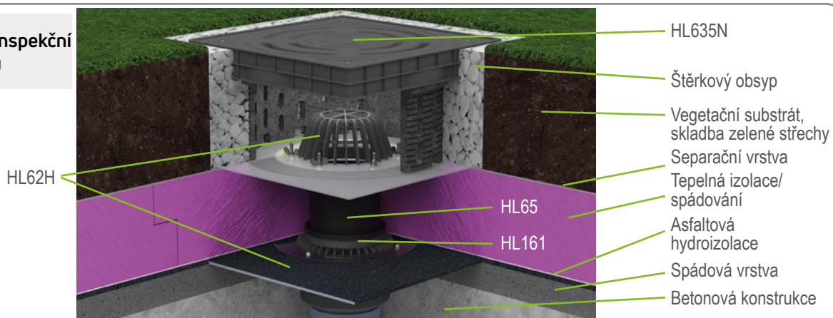
Nouzové odvodnění Intenzivní zeleň s inspekční a drenážní šachtou
