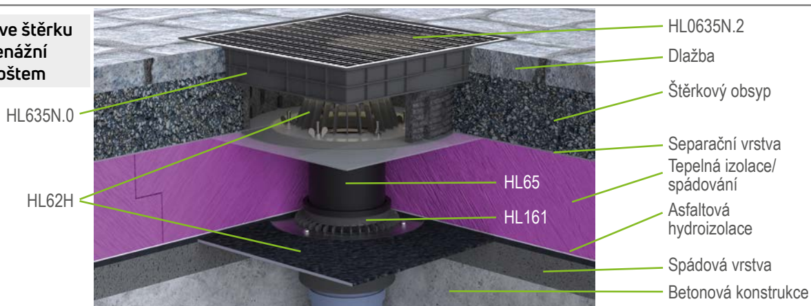
Intenzivní zeleň s inspekční a drenážní šachtou
