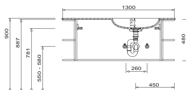
Umyvadlo Odkládací plocha vlevo Výška spodní skříňky 480 mm
