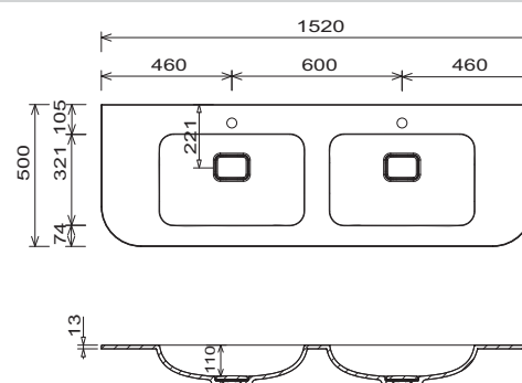
Nábytkové umyvadlo WMS 263R 61
