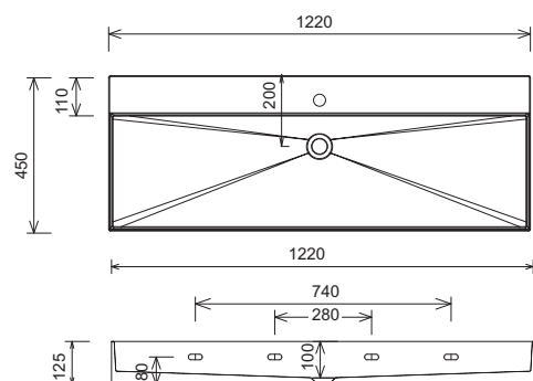
SQUARED WTM 4812 / WTO 4812 Náčrt otvoru pro výřez armatury
