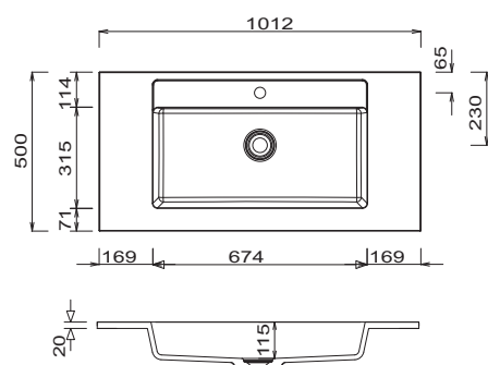
STONEPLUS - umyvadlo 1012 mm
