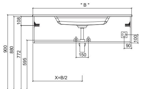
Siena Umyvadlo Výška skříňky pod umyvadlo 320 mm & 360 mm
