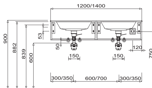
Ibiza Dvojité umyvadlo Výška skříňky pod umyvadlo 240 mm
