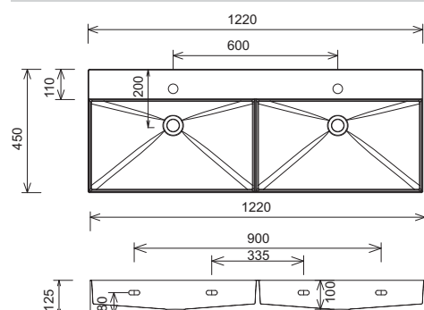
SQUARED WTM 482D / WTO 482D Náčrt otvoru pro výřez armatury
