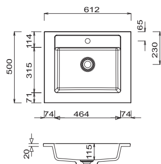
STONEPLUS - umyvadlo 612 mm
