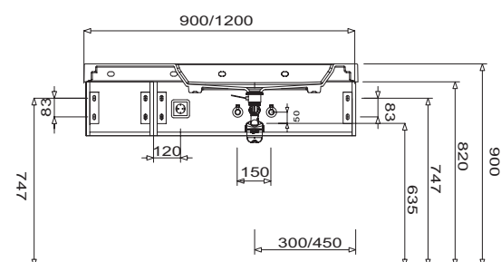
Q!flat Odkládací plocha vlevo Výška skříňky pod umyvadlo 240 mm & 280 mm
