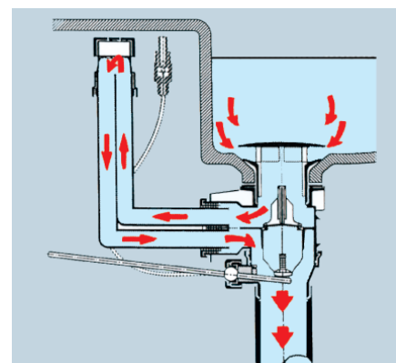
3. Vypouštěcí ventil - otevřený
