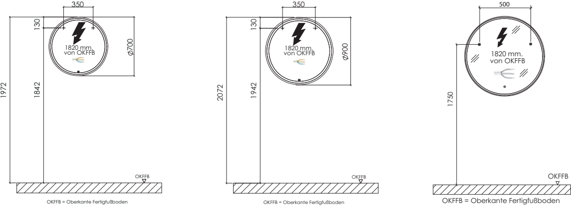
FSR 4070 01 FSR 4090 01 FSR 5x80 01
