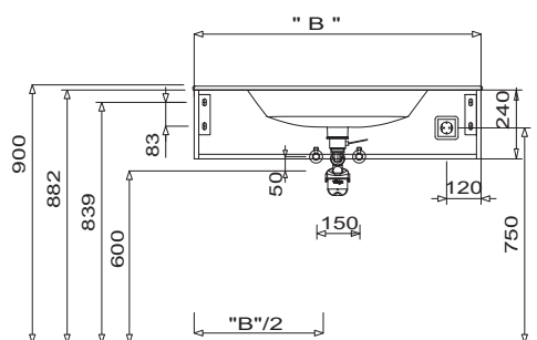
Ibiza Umyvadlo Výška skříňky pod umyvadlo 240 mm
