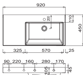
Q!flat 920 - odkládací plocha vlevo
