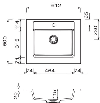
Straight Šířka 612 mm
