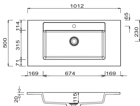
Straight Šířka 1012 mm
