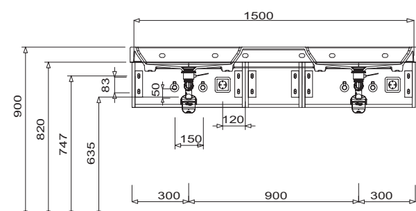
Q!flat Dvojité umyvadlo 1500 mm Výška skříňky pod umyvadlo 240 mm & 280 mm
