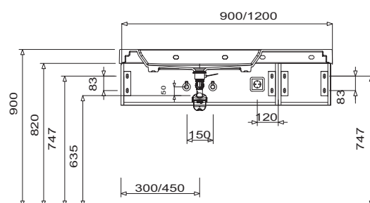
Q!flat Odkládací plocha vpravo Výška skříňky pod umyvadlo 240 mm & 280 mm
