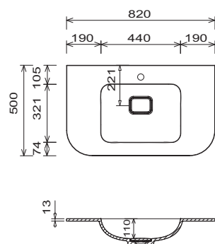
Nábytkové umyvadlo WMS 2608 61
