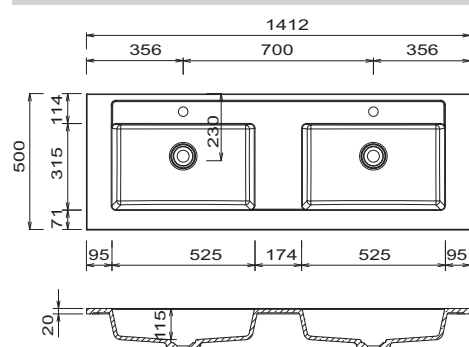
STONEPLUS - umyvadlo 1412 mm
