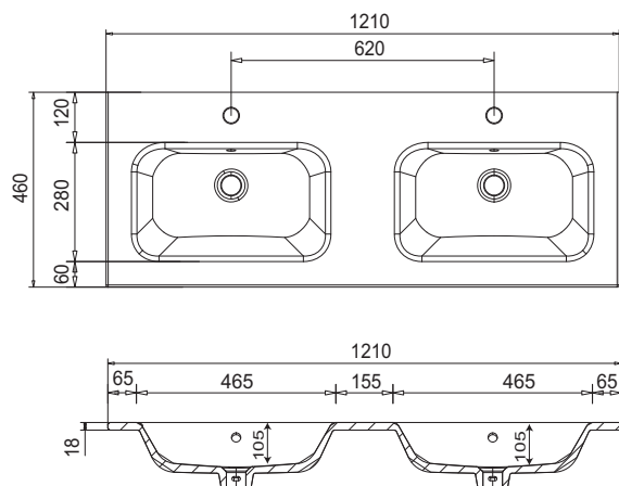
Cuba 1210 Dvojité umyvadlo
