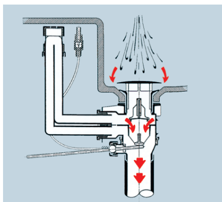
1. Vypouštěcí ventil - otevřený
