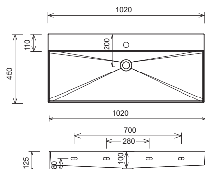
SQUARED WTM 4810 / WTO 4810 Náčrt otvoru pro výřez armatury
