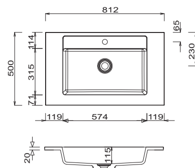
STONEPLUS - umyvadlo 812 mm
