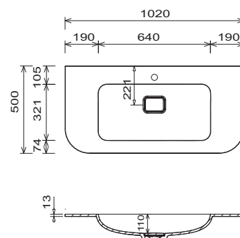
Nábytkové umyvadlo WMS 2610 61
