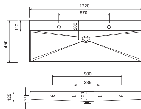
WTM 4822 1 / WTO 4812 1 Náčrt otvoru pro výřez armatury
