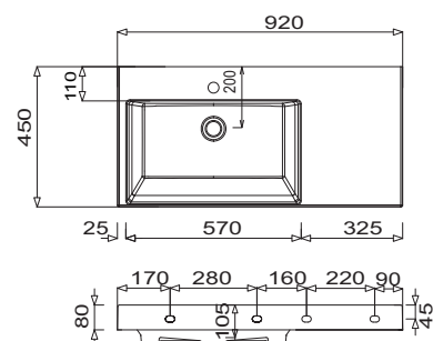
Q!flat 920 - odkládací plocha vpravo
