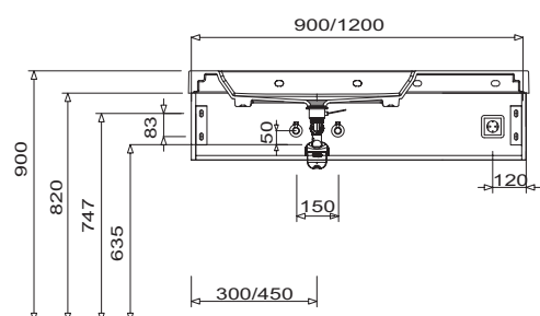
Q!flat Odkládací plocha vpravo Výška skříňky pod umyvadlo 240 mm & 280 mm
