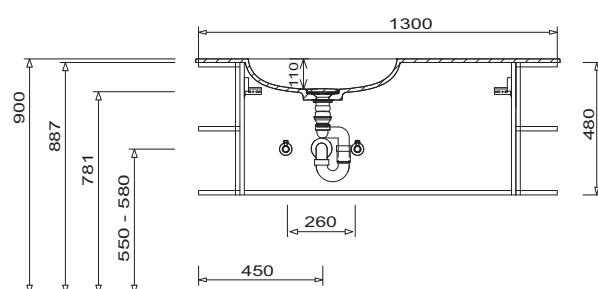
Umyvadlo Odkládací plocha vpravo Výška spodní skříňky 480 mm
