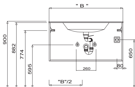
Ibiza Umyvadlo Výška skříňky pod umyvadlo 480 mm, 520 mm, 560 mm, 640 mm & 720
