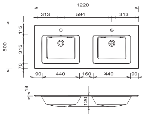
Ibiza 1220 Dvojité umyvadlo
