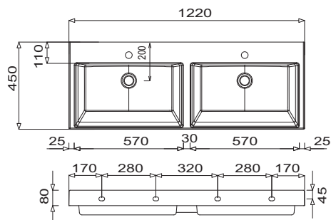
Q!flat 1220 Dvojité umyvadlo
