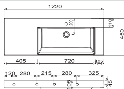
Q!flat 1220 - odkládací plocha vlevo
