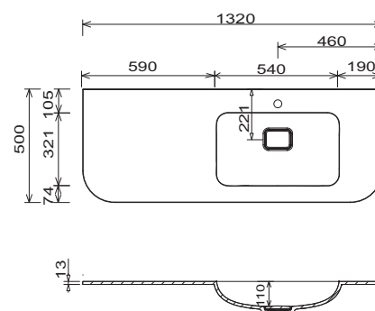
Nábytkové umyvadlo WMS 263L 61
