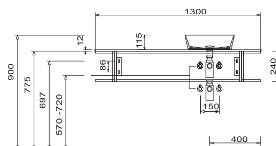
Přídavné umyvadlo Odkládací plocha vlevo Výška skříňky pod umyvadlo 240 mm Výška umyvadla odpovídá výšce umyvadla Nizza kulatý
