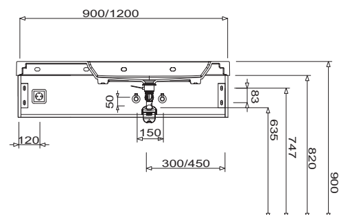
Q!flat Odkládací plocha vlevo Výška skříňky pod umyvadlo 240 mm & 280 mm
