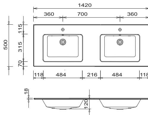
Ibiza 1420 Dvojité umyvadlo
