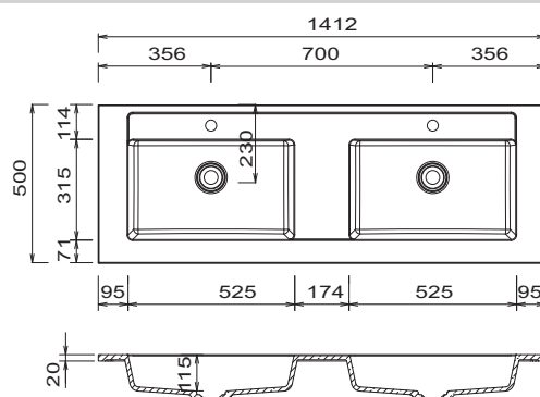
Dvojité umyvadlo Straight Šířka 1412 mm
