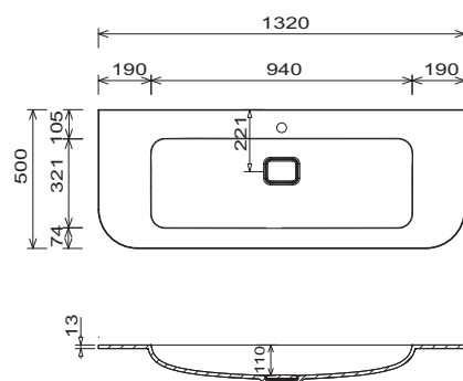
Nábytkové umyvadlo WMS 2613 61
