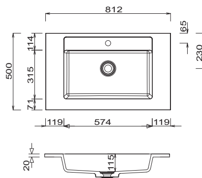
Straight Šířka 812 mm
