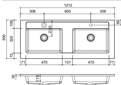
Dvojité umyvadlo Straight Šířka 1212 mm
