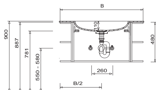
Umyvadlo Výška spodní skříňky 480 mm
