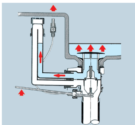
2. Vypouštěcí ventil - uzavřený
