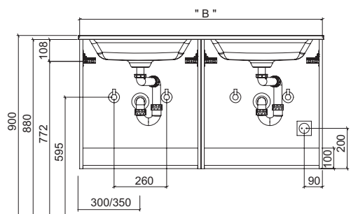
Siena Dvojité umyvadlo Výška skříňky pod umyvadlo 480 mm, 520 mm, 560 mm, 640 mm & 720
