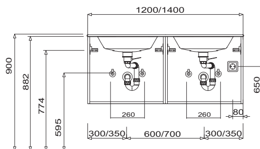
Ibiza Dvojité umyvadlo Výška skříňky pod umyvadlo 480 mm, 520 mm, 560 mm, 640 mm & 720
