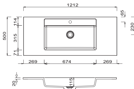
Straight Šířka 1212 mm
