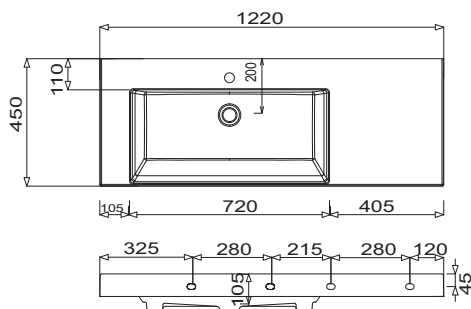
Q!flat 1220 - odkládací plocha vpravo
