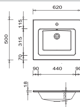
KERAMICKÉ umyvadlo 620 mm
