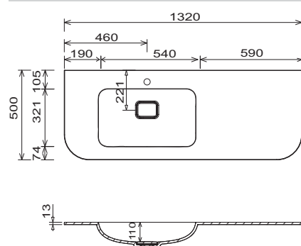
Nábytkové umyvadlo WMS 263R 61
