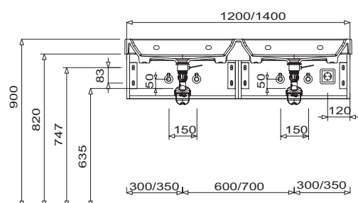
Q!flat Dvojité umyvadlo 1200 mm & 1400 mm Výška skříňky pod umyvadlo 240 mm & 280 mm
