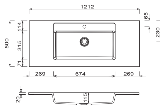
STONEPLUS - umyvadlo 1212 mm
