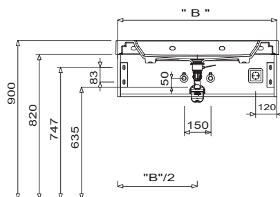
Q!flat Umyvadlo Výška skříňky pod umyvadlo 240 mm & 280 mm
