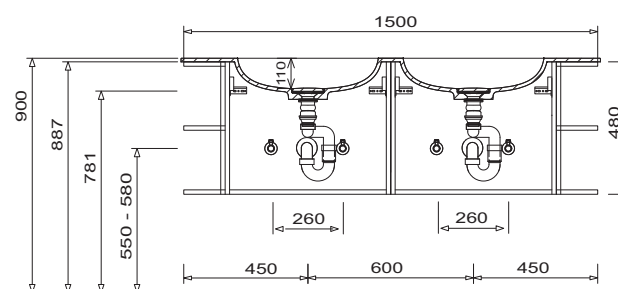
Dvojité umyvadlo Výška spodní skříňky 480 mm
