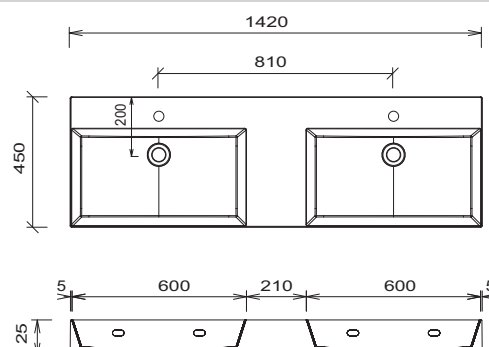
SQUARED WTM 484D / WTO 484D Náčrt otvoru pro výřez armatury
