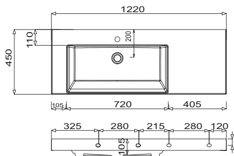
Q!flat 1220 - odkládací plocha vpravo
