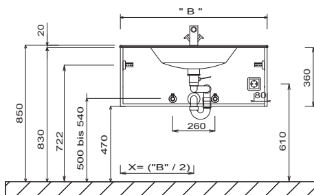
Jednodílné umyvadlo - výška spodní skříňky 360 mm Výška umyvadla odpovídá výšce umyvadla Stoneplus
