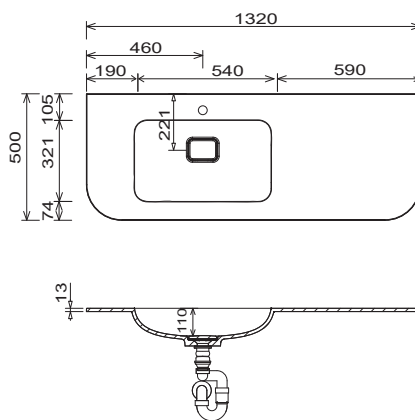
Nábytkové umyvadlo WMS 263R 61
