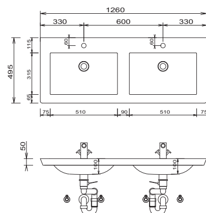
Valencia 1060 Dvojité umyvadlo
