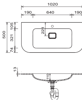
Nábytkové umyvadlo WMS 2610 61
