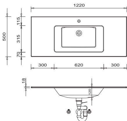
KERAMICKÉ umyvadlo 1220 mm
