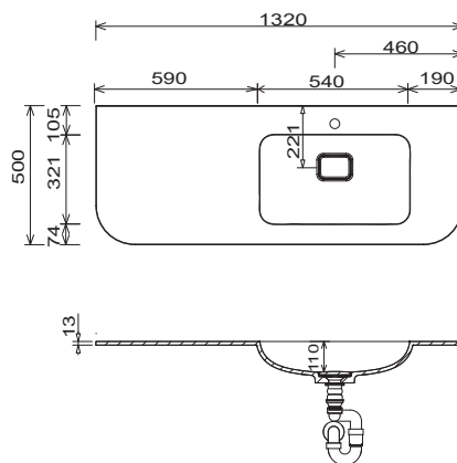
Nábytkové umyvadlo WMS 263L 61
