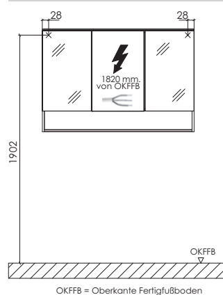
Elektrické přípojky pro zrcadlovou skříňku
