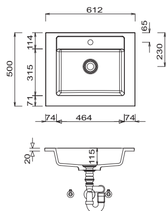
STONEPLUS - umyvadlo 612 mm
