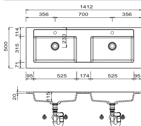
STONEPLUS - umyvadlo 1412 mm
