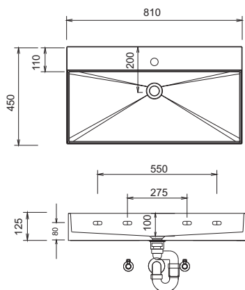
SQUARED WTM 4808 / WTO 4808 Náčrt otvoru pro výřez armatury
