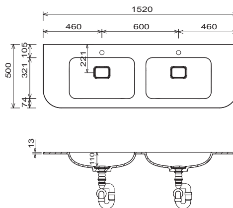
Nábytkové umyvadlo WMS 263R 61
