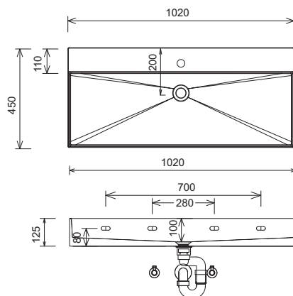
SQUARED WTM 4810 / WTO 4810 Náčrt otvoru pro výřez armatury
