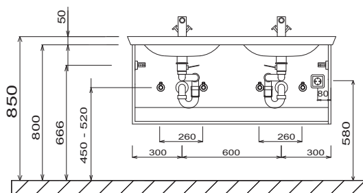
Dvojité umyvadlo Valencia Skříňka pod umyvadlo bez úchyty
