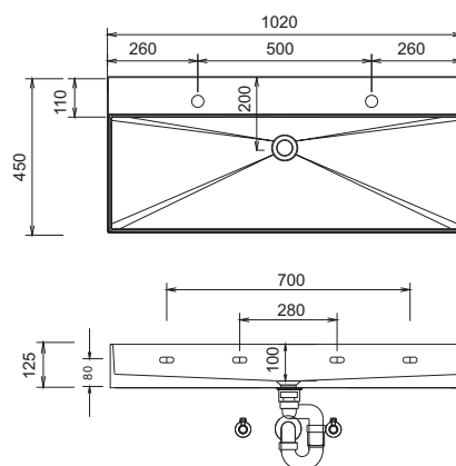
WTM 4821 1 / WTO 4810 1 Náčrt otvoru pro výřez armatury
