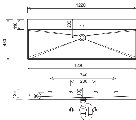
SQUARED WTM 4812 / WTO 4812 Náčrt otvoru pro výřez armatury
