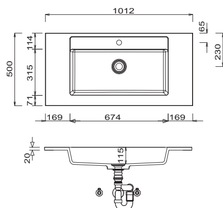
STONEPLUS - umyvadlo 1012 mm
