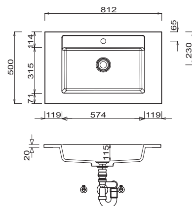
STONEPLUS - umyvadlo 812 mm
