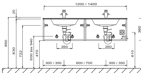
Dvojumyvadlo - výška spodní skříňky 360 mm Výška umyvadla odpovídá výšce umyvadla Stoneplus
