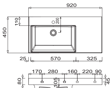
Q!flat 920 - odkládací plocha vpravo
