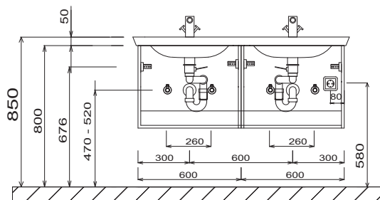
Dvojité umyvadlo Valencia Skříňka pod umyvadlo s úchytem
