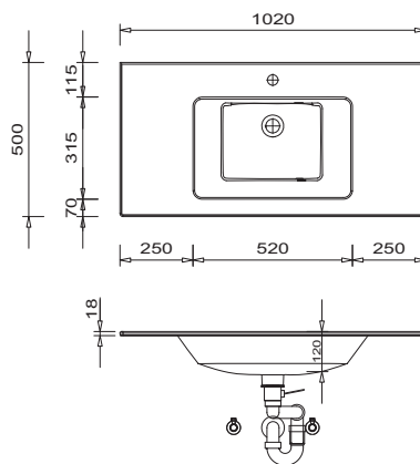
KERAMICKÉ umyvadlo 1020 mm
