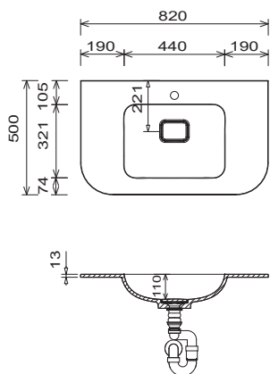
Nábytkové umyvadlo WMS 2608 61
