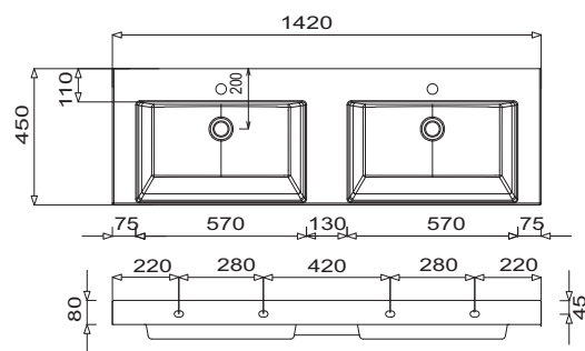
Q!flat 1420 Dvojité umyvadlo
