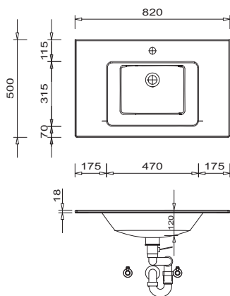
KERAMICKÉ umyvadlo 820 mm
