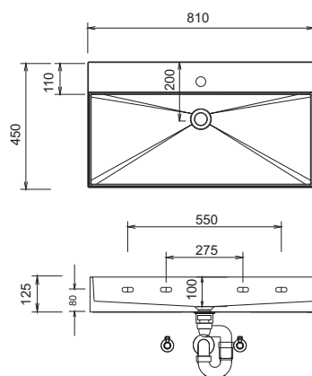
WTM 4808 1 / WTO 4808 1 Náčrt otvoru pro výřez armatury
