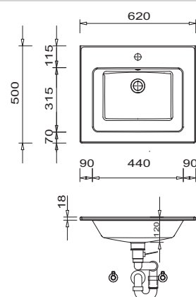
KERAMICKÉ umyvadlo 620 mm
