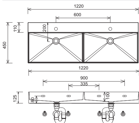
SQUARED WTM 482D / WTO 482D Náčrt otvoru pro výřez armatury
