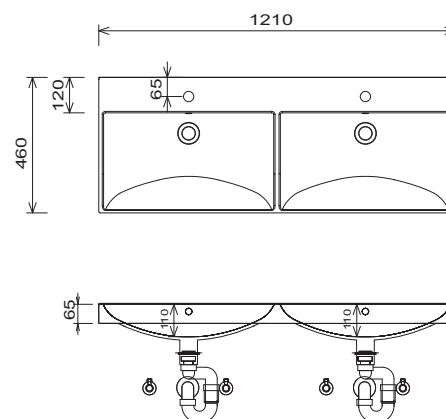
K-Line 1210 Dvojité umyvadlo
