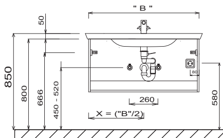
Umyvadlo Valencia Skříňka pod umyvadlo bez úchyty
