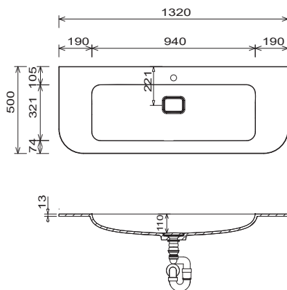
Nábytkové umyvadlo WMS 2613 61
