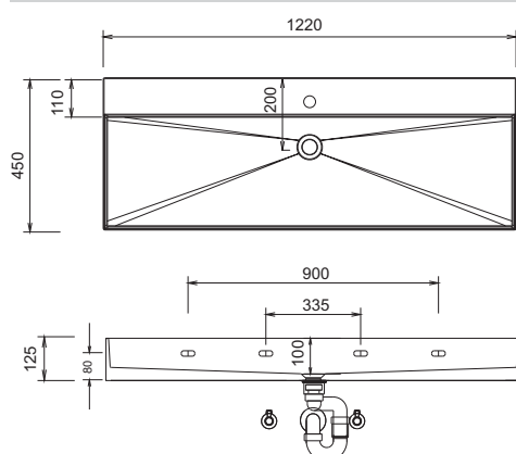
WTM 4812 1 / WTO 4812 1 Náčrt otvoru pro výřez armatury
