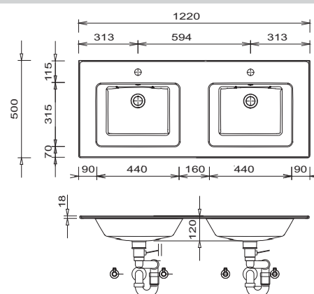
Ibiza 1220 Dvojité umyvadlo
