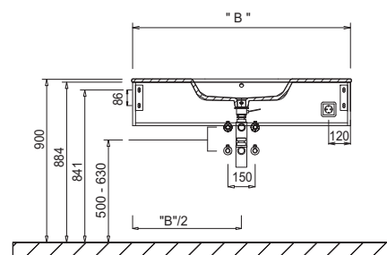
Cuba Umyvadlo Výška skříňky pod umyvadlo 240 mm & 280 mm
