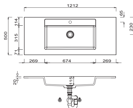
STONEPLUS - umyvadlo 1212 mm
