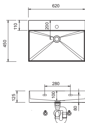
WTM 4806 1 / WTO 4806 1 Náčrt otvoru pro výřez armatury
