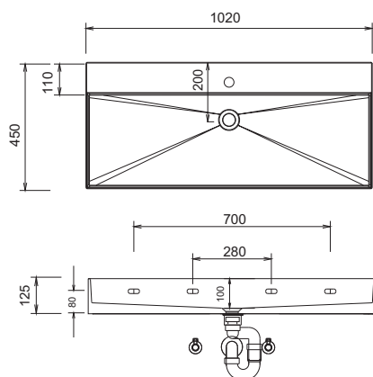
WTM 4810 1 / WTO 4810 1 Náčrt otvoru pro výřez armatury
