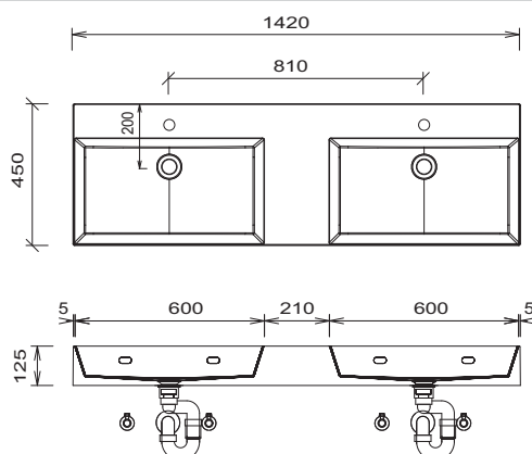
SQUARED WTM 484D / WTO 484D Náčrt otvoru pro výřez armatury
