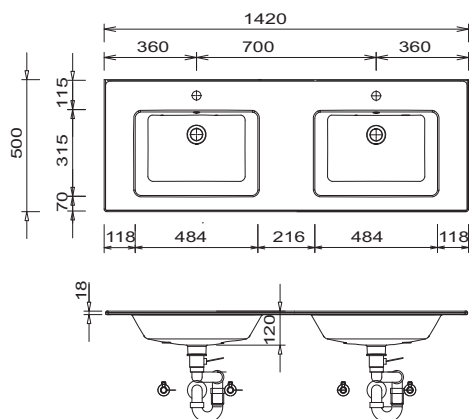
KERAMICKÉ umyvadlo 1420 mm
