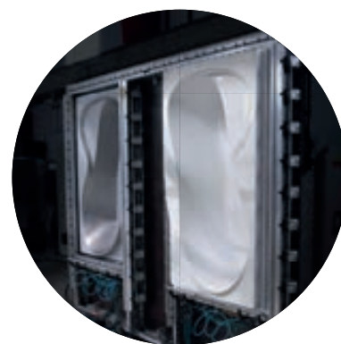
Lisovna RAVAK Vznik akrylátového výlisu budoucí vany pomocí technologie svislého ohřevu.
