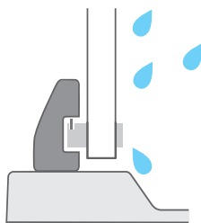
Rám ve spodní části koutu: Nexty, Pivot, Blix Slim, Blix, Blix II, Supernova
