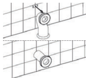
Vario odpad umožňující vodorovné nebo svislé napojení
