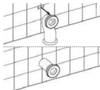
Vario odpad umožňující vodorovné nebo svislé napojení
