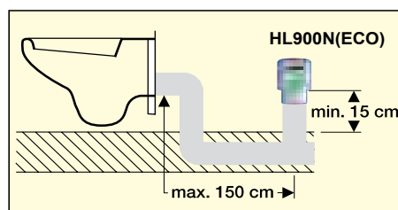
Obr. 3 Přívzdušňovací ventil pro WC na ležatém připojovacím potrubí
