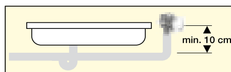
Obr. 2 Přívzdušňovací ventil pro sprchovou vaničku na ležatém připojovacím potrubí
