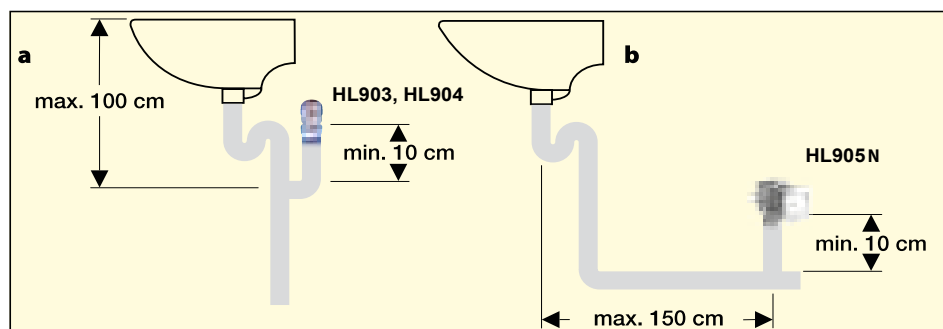
Obr. 1 Přívzdušňovací ventil u umyvadla a – na svislé části připojovacího potrubí; b – na ležaté části připojovacího potrubí
