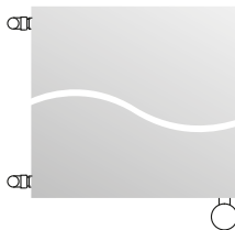
[Obr. 5 - připojení topné tyče přímo do radiátoru ÚT s bočním připojením k instalaci.] Připojení L8, P1, S8, Y1
